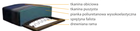
K - pianka wysokoelastyczna
