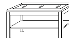
Stolik przeszklony z półką 1050 x 600 x 550
