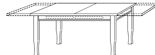
Stół rozkładany 1500 (2500) x 900 x 760
