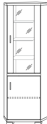
Witryna narożna 860 x 610 x 610 x 2040
